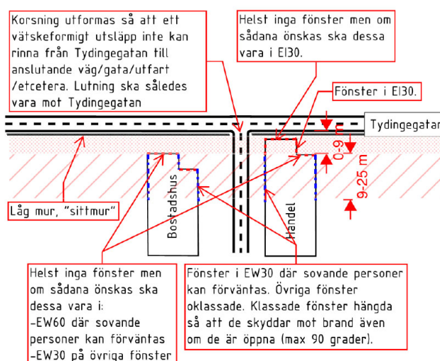
Figur 7. Illustration över aktuella riskreducerande åtgärder intill Tydingegatan/väg 119.
